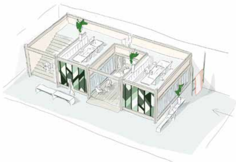
Sopra: assonometria della struttura principale con i diversi ambienti e il soppalco aperto al piano superiore. Sotto e in basso a destra: dettaglio del telaio di legno che incornicia il tessuto a maglia Kvadrat Cilos, sulla sinistra una scaffalatura lungo la parete raccoglie il catalogo tessile
